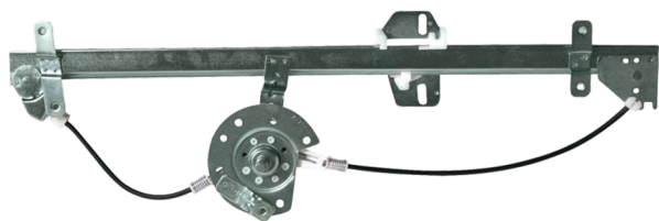
R-2314 E/D Máquina Reguladora 1938 S / Atego / Axor - Pino Longo N° Orig. 973.720.01.46 (LE) / 973.720.02.46 (LD)
