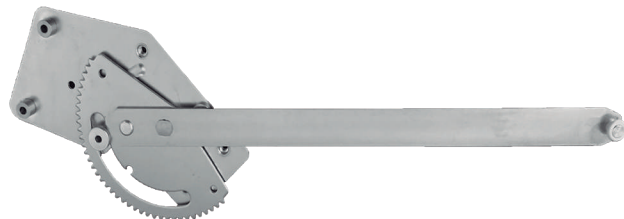
R-2126 E/D Máquina Reguladora HPN 709 / 1935 1991...2000 - 12/24V C/ Motor - S/ Motor Fixação Motor Mabuchi - (Motor invertido) N° Orig. A384.720.70.46 (LE) / A384.720.71.46 (LD)
