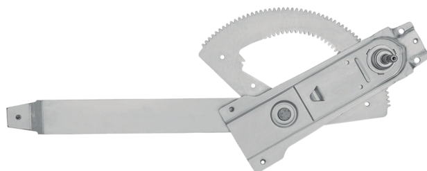
R-5149 E/D Máquina Reguladora F-4000 Sapão 1992...1999 N° Orig. T71.837.501.D (LE) / T71.837.502.D (LD)
