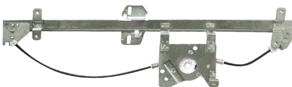
R-2310 E/D Máquina Reguladora 1938 S / Atego / Axor C/ Motor - S/ Motor Fixação Motor Original N° Orig. 979.720.03.46 (LE) / 979.720.04.46 (LD)
