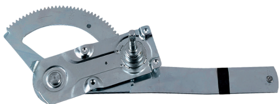
R-2305 E/D Máquina Reguladora Alemão - Exportação N° Orig. N/A (LE) / N/A (LD)
