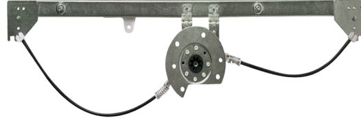
R-2311 E/D Máquina Reguladora Accelo 715 - 12V / 915 - 24V ...2011 C/ Motor - S/ Motor Fixação Motor Mabuchi - (Motor invertido) N° Orig. 979.720.01.46 SM (LE) / 979.720.02.46 SM (LD) 12V N° Orig. 979.720.70.46 SM (LE) / 979.720.71.46 SM (LD) 24V
