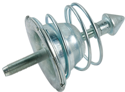
F-2306 S Fecho do capô superior HPN 2001... N° Orig. A-694.880.01.60
