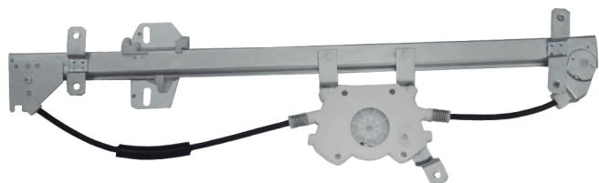
R-2312 E/D Máquina Reguladora 1938 S / Atego / Axor - 24V C/ Motor - S/ Motor Fixação Motor Mabuchi - (Motor invertido) N° Orig. 979.720.03.46 (LE) / 979.720.04.46 (LD)
