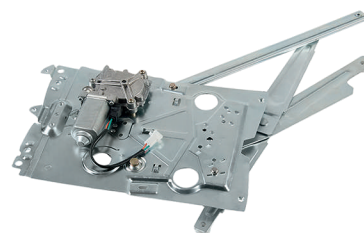
R-2615 E/D Máquina Reguladora FH12 / FH13 / FM 1994... 24V C/ Motor - S/ Motor Fixação Motor Original - Todos N° Orig. 3.176.545 (LE) / 3.176.546 (LD)
