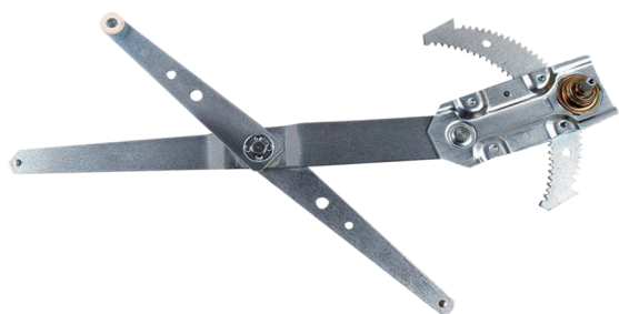
R-5148 E/D Máquina Reguladora Cargo 1981... N° Orig. 81DBE23201AJ (LE) / 81DBE23200AJ (LD)
