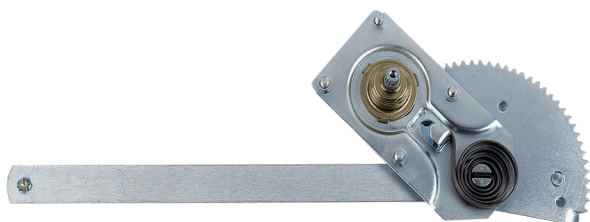
R-2605 E/D Máquina Reguladora LK 140 / 141 1988... N° Orig. 187.719 (LE) / 187.720 (LD)
