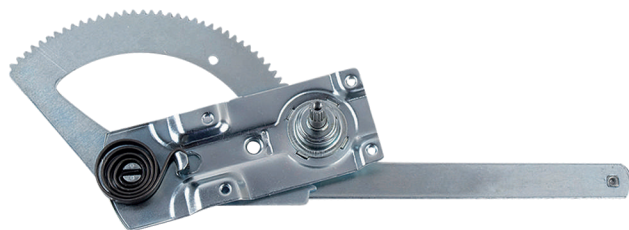
R-2122 E/D Máquina Reguladora 1111-1113-1313-1513-2013- 2213 1983...1990 Pino Longo N° Orig. 331.725.70.02 (LE) / 331.725.71.02 (LD)
