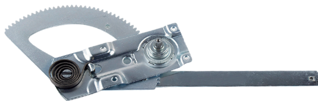
R-2121 E/D Máquina Reguladora 1111-1113-1313-1513-2013- 2213 1973...1982 Pino Curto N° Orig. 344.768.00.01 (LE) / 344.768.01.01 (LD)
