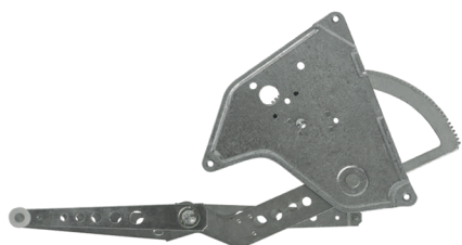
R-2608 E/D Máquina Reguladora Série 3 / R112 / R113 / T112 / T113 1981...1997 24V C/ Motor - S/ Motor Fixação Motor Original N° Orig. 376.673 (LE) / 376.674 (LD)
