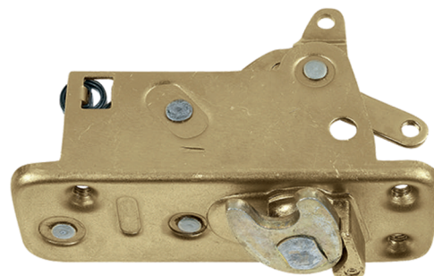
F-2301 E/D Fechadura 1111-1113-1313-1513-2013-2213 ...1990
