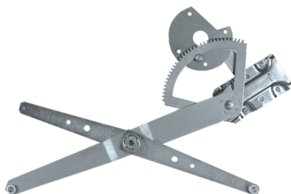
R-5233 E/D Máquina Reguladora Cargo 1981...2013 12/24V C/ Motor - S/ Motor Fixação Motor Mabuchi N° Orig. 81DBE23201AJ (LE) / 81DBE23200AJ (LD)
