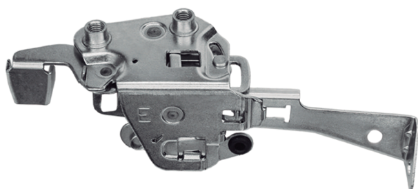
F-2303 E/D Fechadura interna 709 / 909 ...1996
