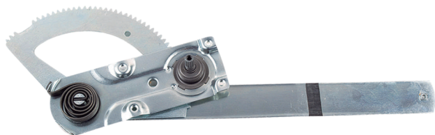
R-2124 E/D Máquina Reguladora MB Zetros / Unimog 1991... Pino Longo - Exportação N° Orig. 381.725.00.02 (LE) / 381.725.01.02 (LD)
